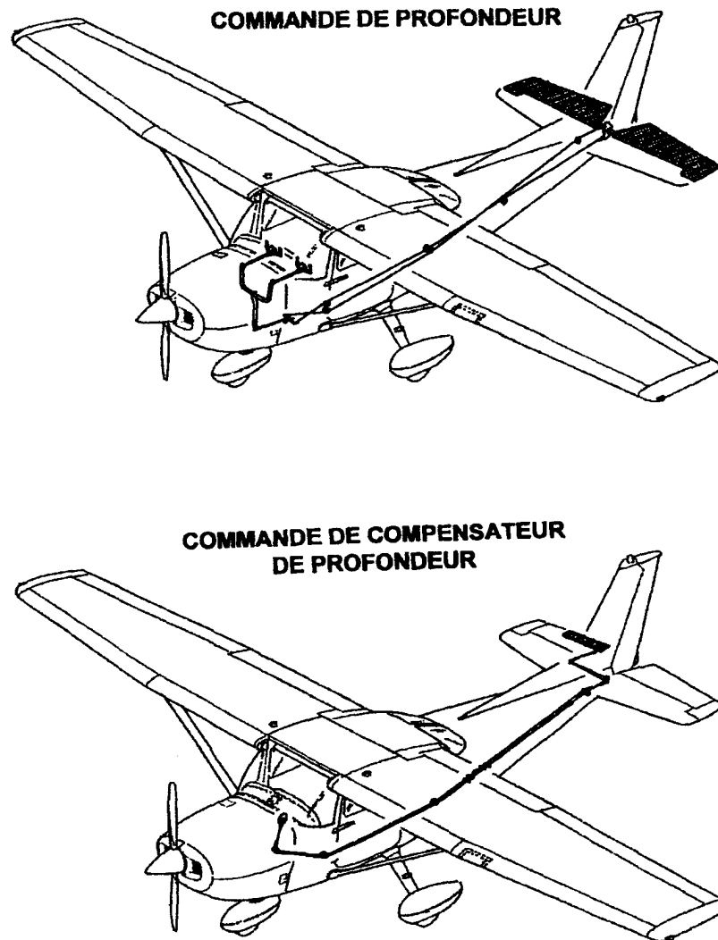
Figure 7-1. Commandes de vol et de compensateurs (2/2)
