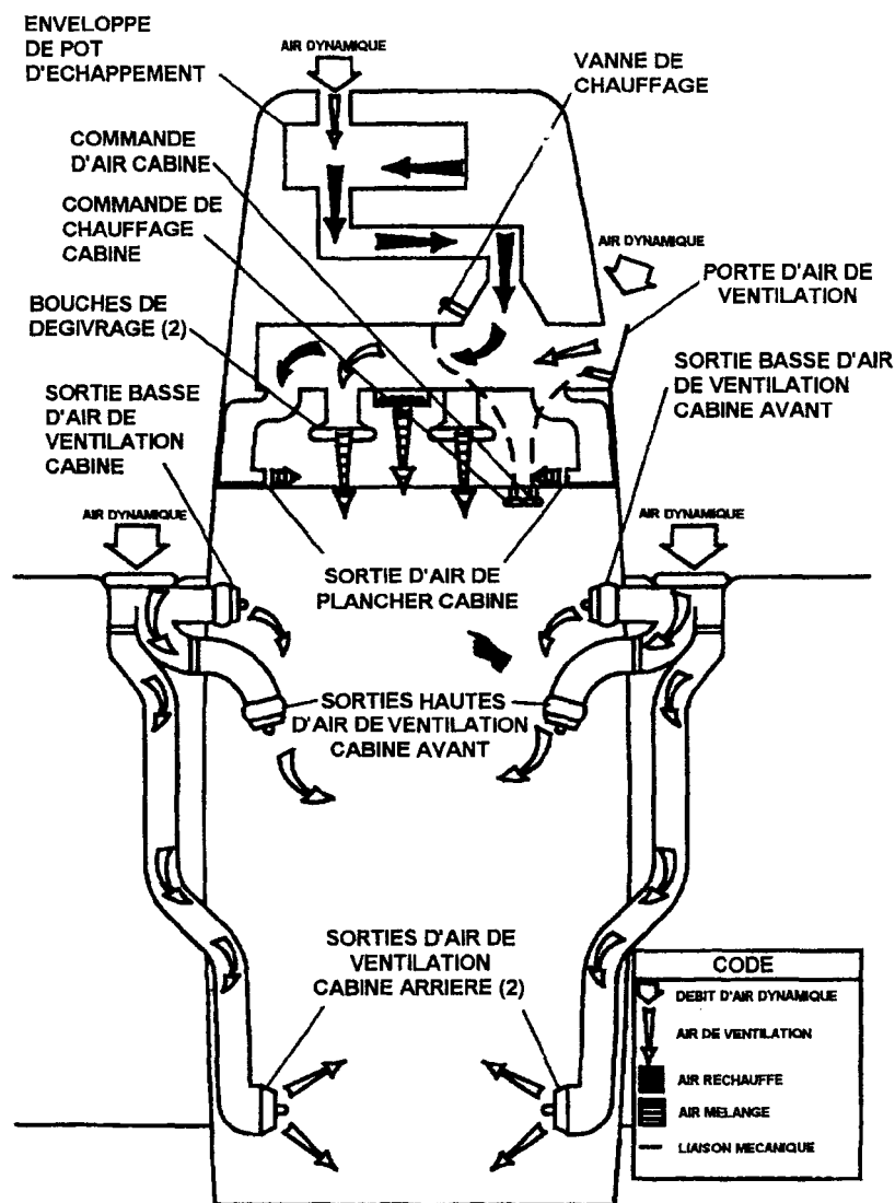
Figure 7-8. Système de chauffage, ventilation et dégivrage
