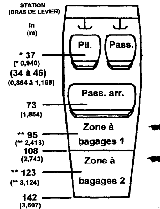
FIGURE 6-3. Schéma d'aménagement
