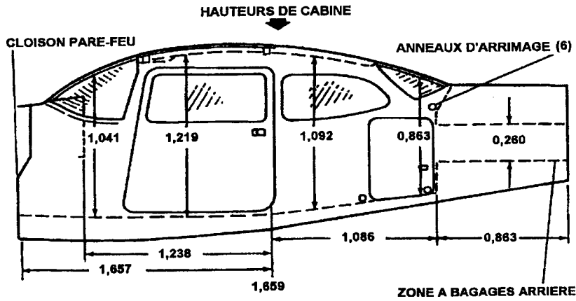
DIMENSIONS DES OUVERTURES DE PORTES
